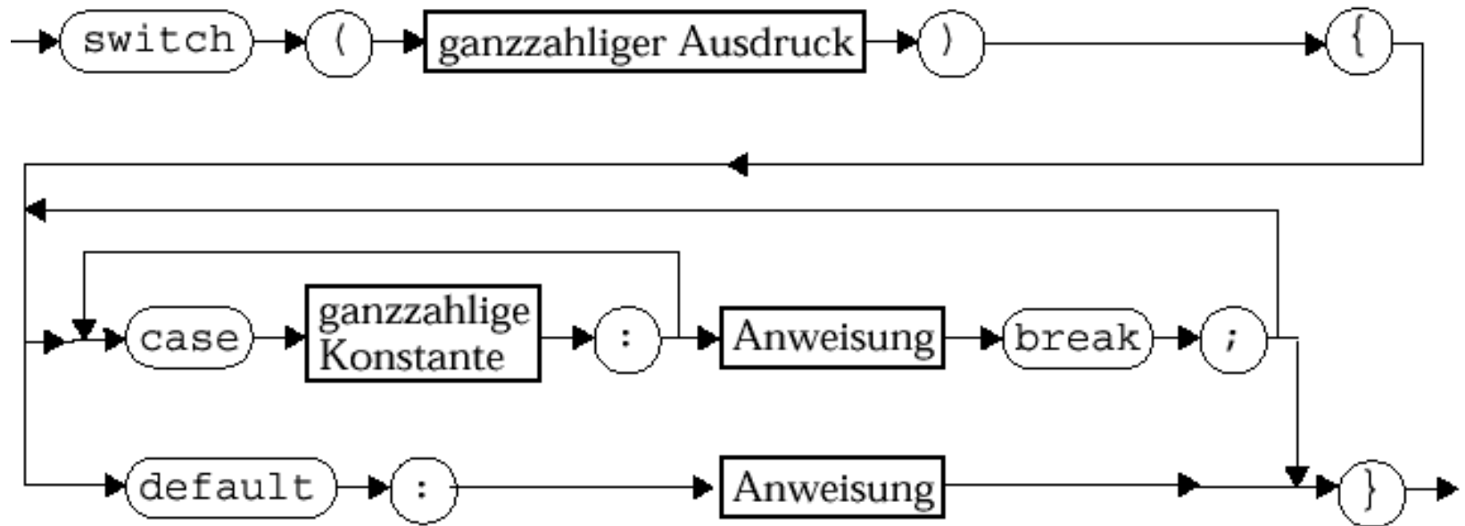
Abb. 2-8 Syntax der switch-Anweisung
